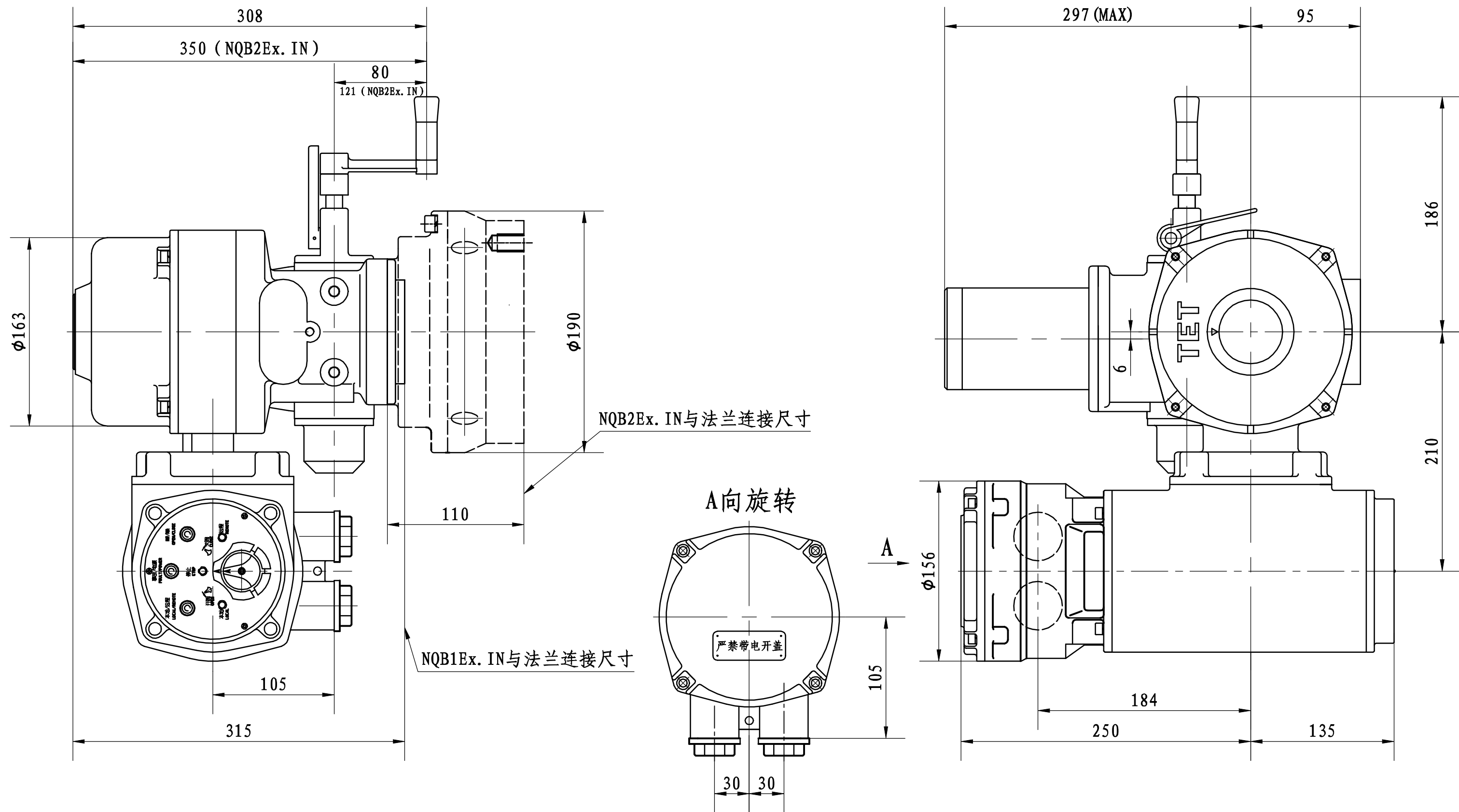
NQB1Ex. IN、NQB2Ex. IN防爆整体型产品外形尺寸图
